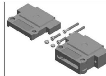
HOOD115 - IDC - XX X Y - L 1 2 3
