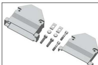
HOOD117 - XX V - L 1 2
