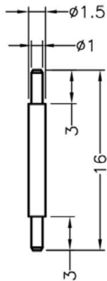
HOLE IN P.C.B \phi 1.0
