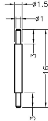
HOLE IN P.C.B \phi 1.0
